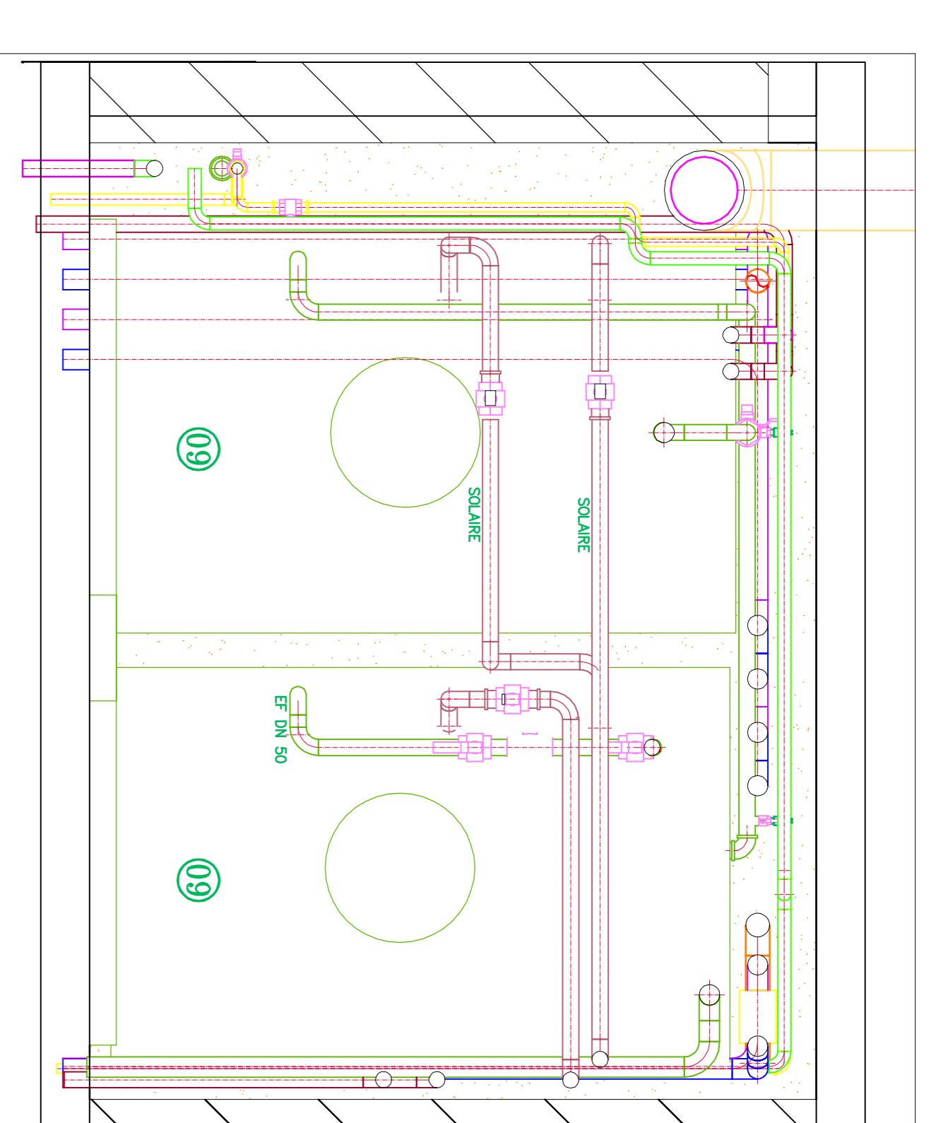
Coupe D-D
